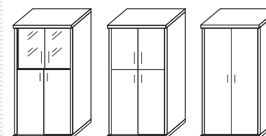
A.СУ-1.7 Л/Пр A.СУ-1.8 Л/Пр A.СУ-1.9 Л/Пр размеры 403x365x1975
